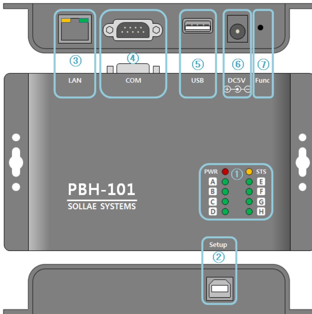
그림 1-2 패널 레이아웃
