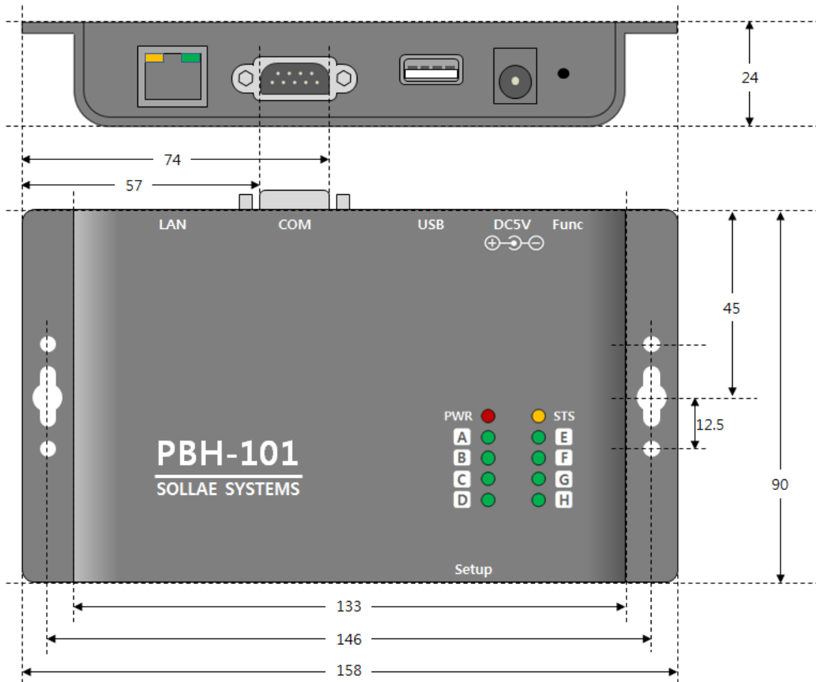
그림 1-1 치수
